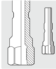
Stecknippel KW : 1/4" IG. Edelstahl. SW 19. Stecknippel für umspritzte Lanzen
