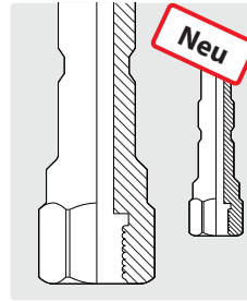
Stecknippel KW : 1/4" IG. Edelstahl poliert. SW 19. Für umspritzte Lanzen. Stecknippel für Aludichtscheiben
